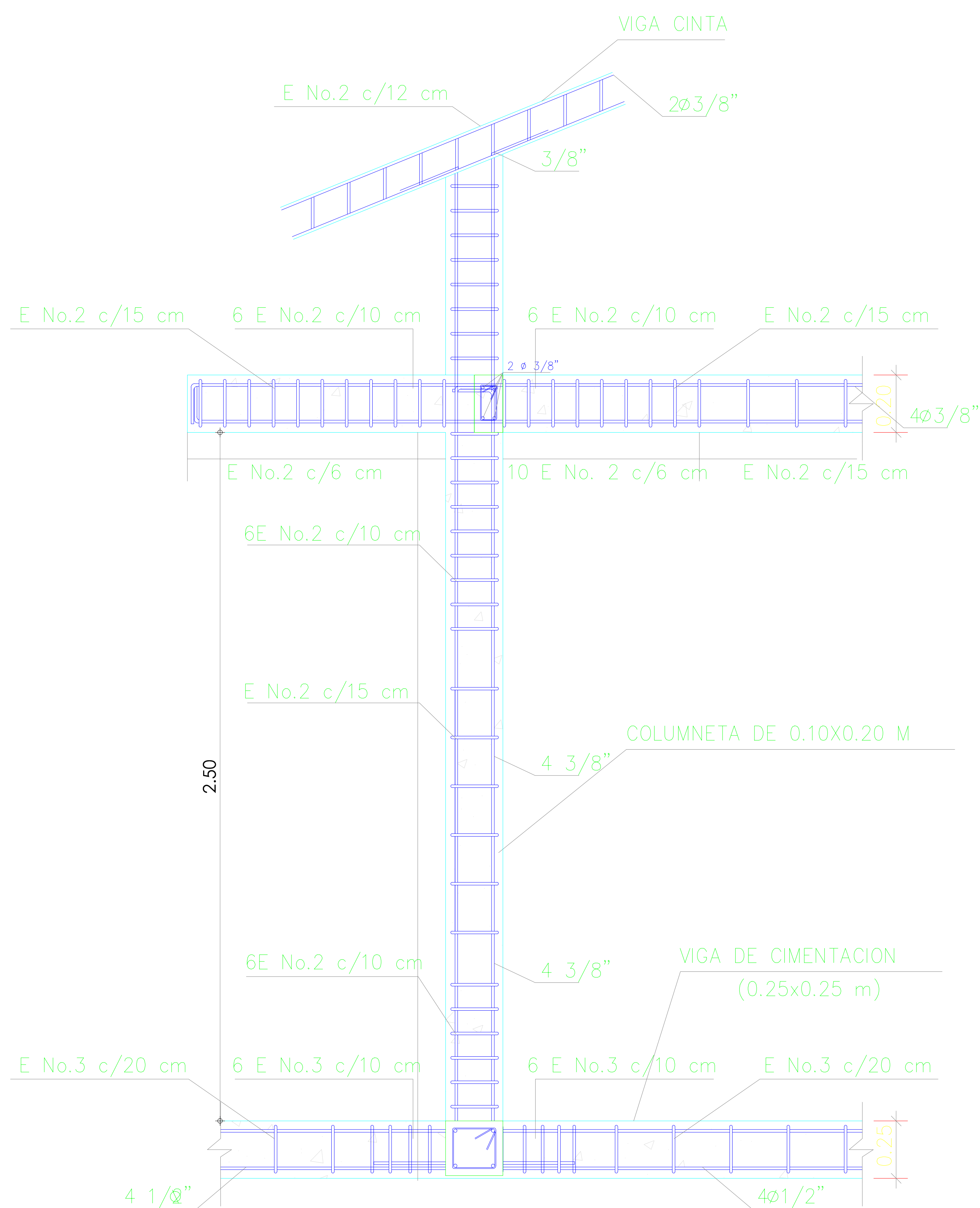
DETALLE ESTRUCTURAL REFUERZO MAMPOSTERIA CONFINADA
