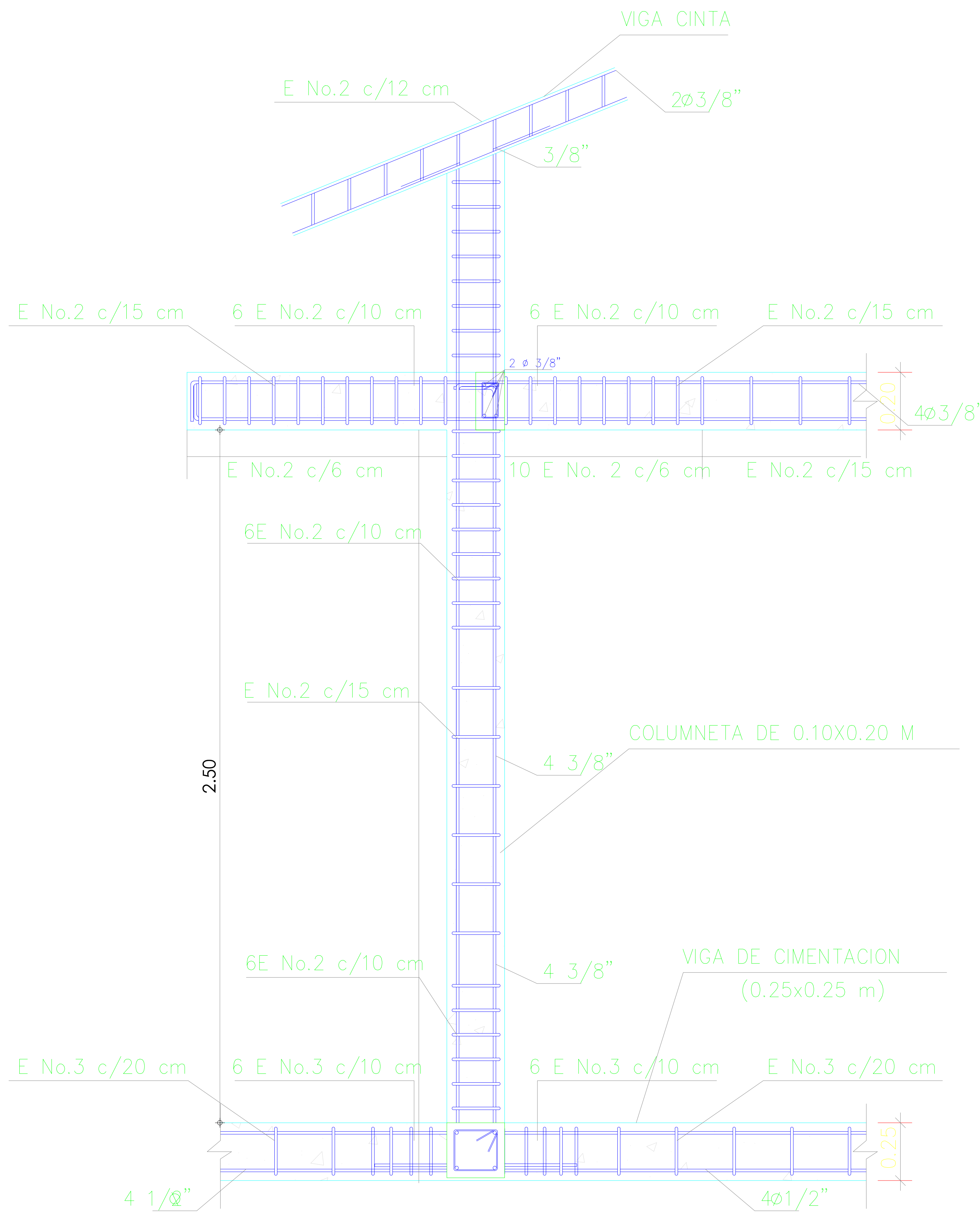
DETALLE ESTRUCTURAL REFUERZO MAMPOSTERIA CONFINADA
