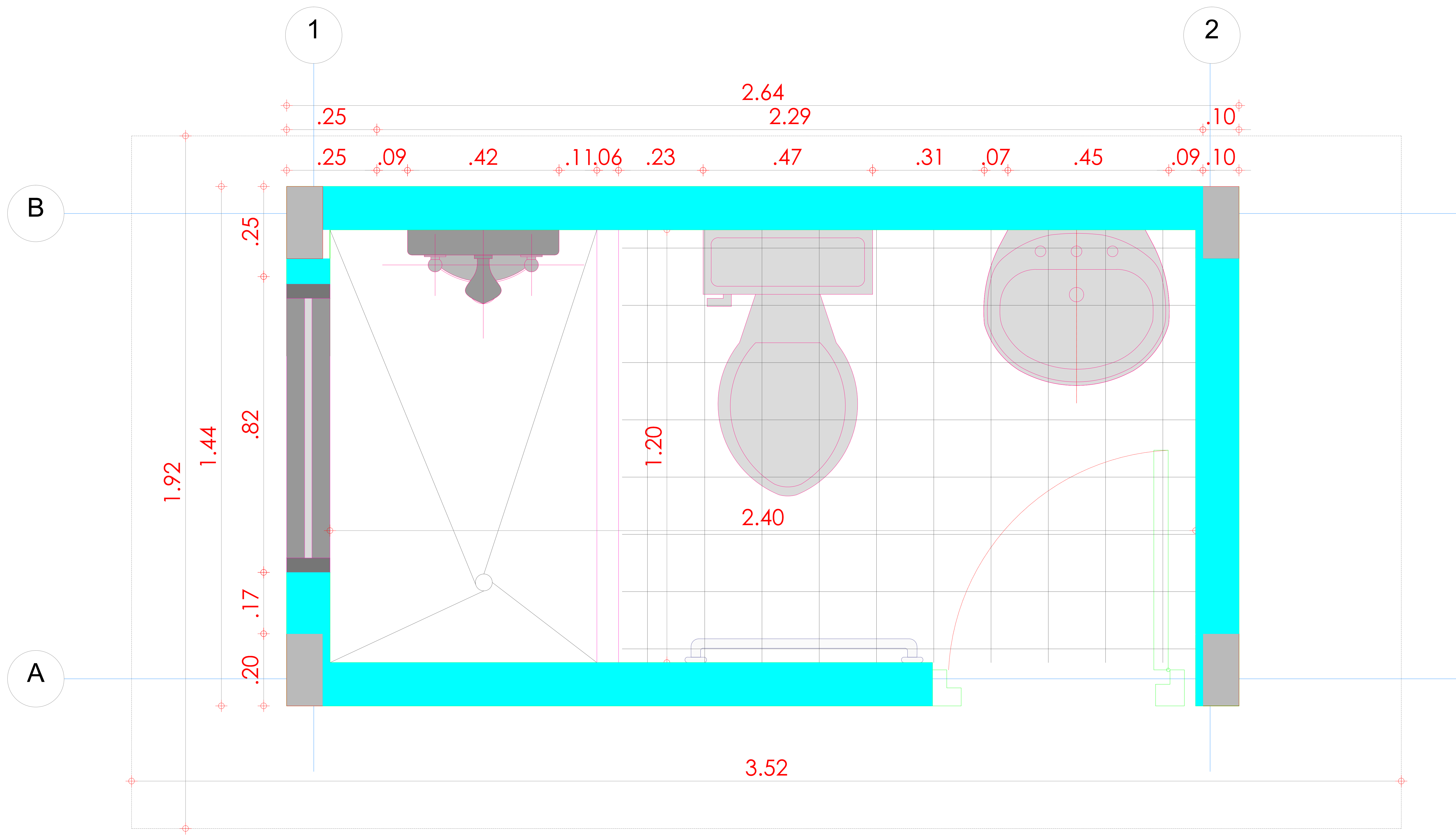
PLANTA ARQUITECTONICA UNIDAD SANITARIA
